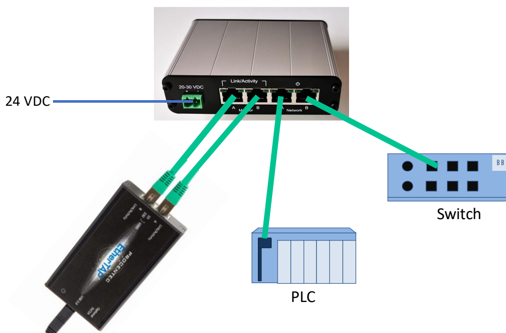
Abbildung 2 - Anschluss des EtherTap an den EtherMIRROR
